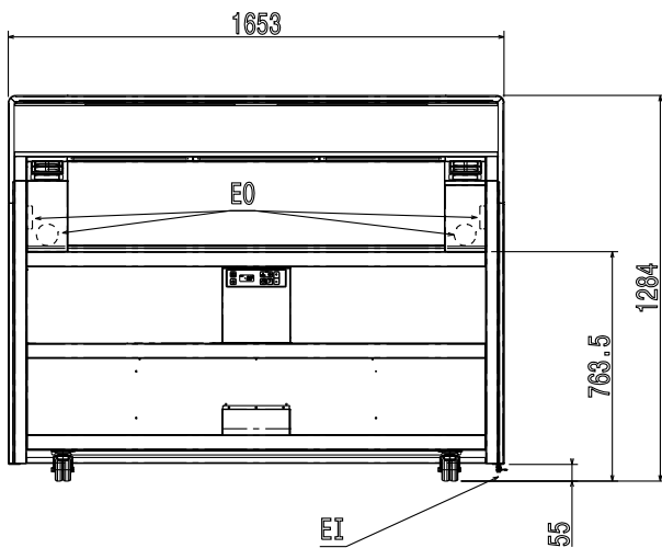
Front aanzicht
