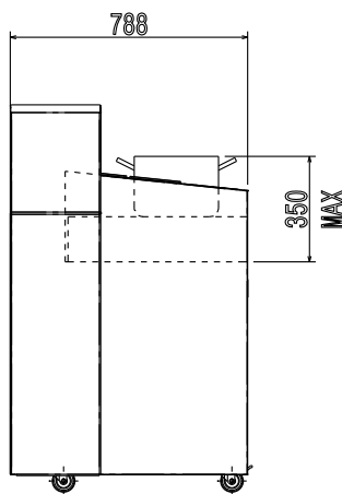
Zij aanzicht
